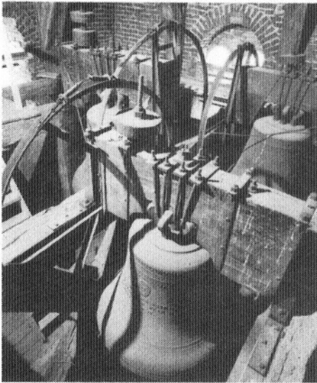
Afb. 5a en 5b: Klokkenstoel en klokken (Coll. RDMZ te Zeist, A.J. v. der Wal, mei 1994).
