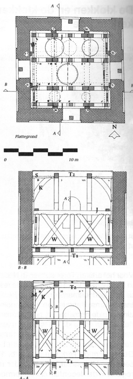
S = sleutelstuk; M = muurstijl; K = korbeel; W = windschoor; J = Juk; T1 = torenverband, eerste laag; T2 = torenverband, tweede laag; N = noord.
