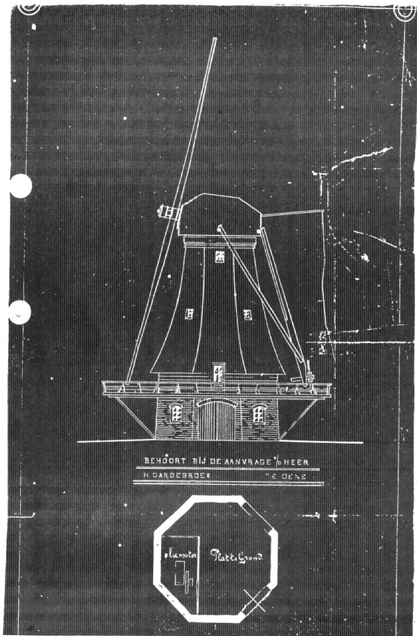
Blauwdruk van de Veldmolen behorend bij de hinderwetaanvraag voor het plaatsen van de petroleummotor door Gardenbroek in 1910.
