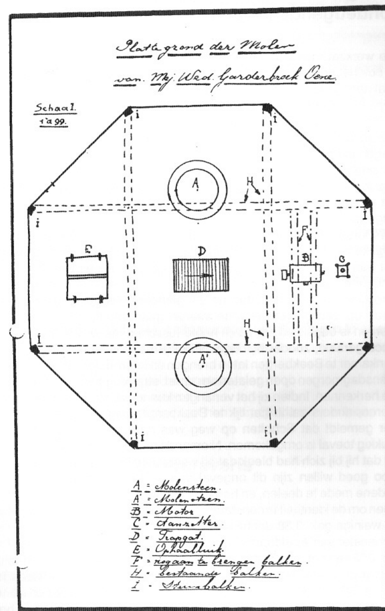
Plattegrondtekening van de Veldmolen behorend bij de hinderwetaanvraag door de weduwe Gardenbroek voor het plaatsen van een elektromotor in 1926. Blijkbaar zou de motor op de steenzolder worden geplaatst.
