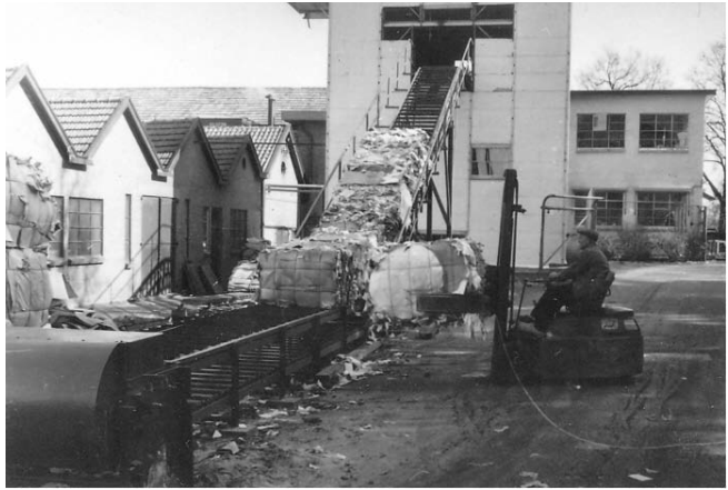
Transportband voor oud papier van de voormalige Bordpapierfabriek Van Delden in 1965. Foto: Hent van Delden
