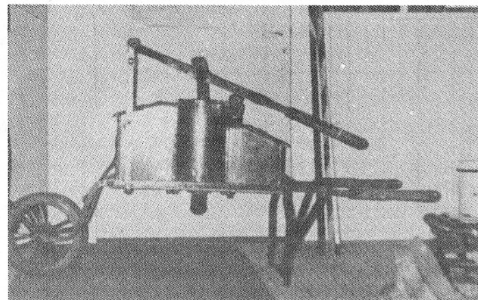
Een ééncylinder huisbrandspuitje naar Kruiwagen model uit + 1750. Aan de afwerking is al te zien, dat de tijd 50 jaar verder is.
